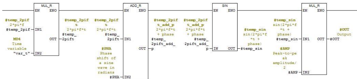
Sl. 3.26. Funkcija „Sine wave“ (2. dio)
