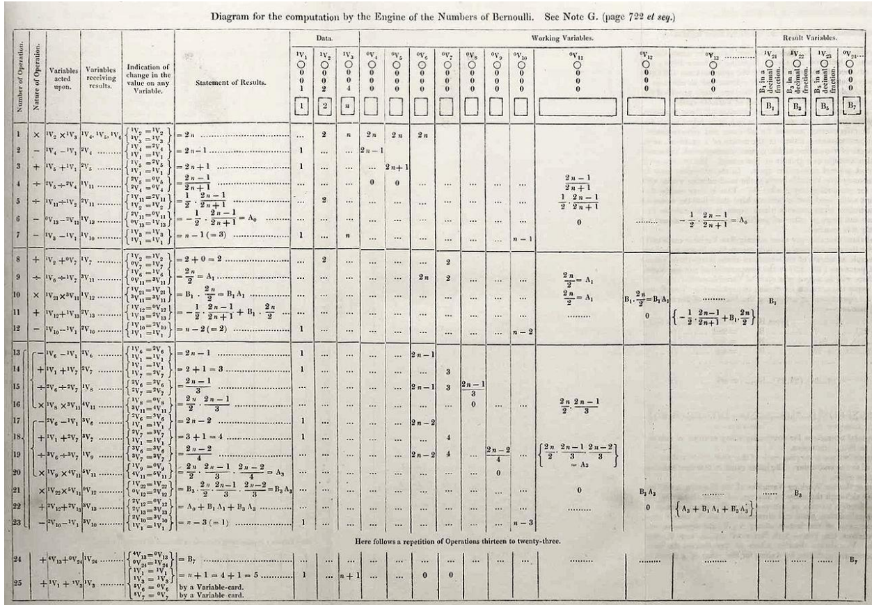
Sl. 4.2. Dijagram za izračun četvrtog Bernoullijevog broja B_7 analitičkim strojem pomoću algoritma Ade Lovelace [6]
