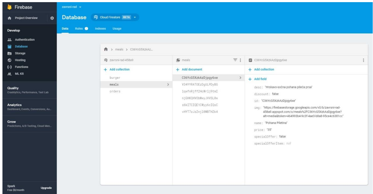
Slika 3.9. Firebase sučelje.
