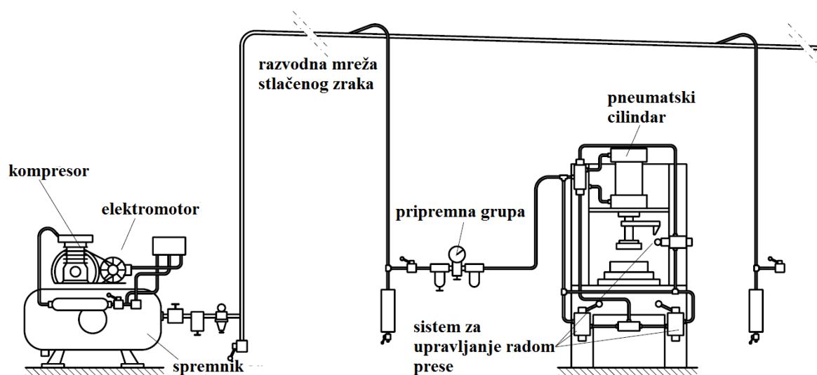
Slika 5.5 – Pneumatski sistem
