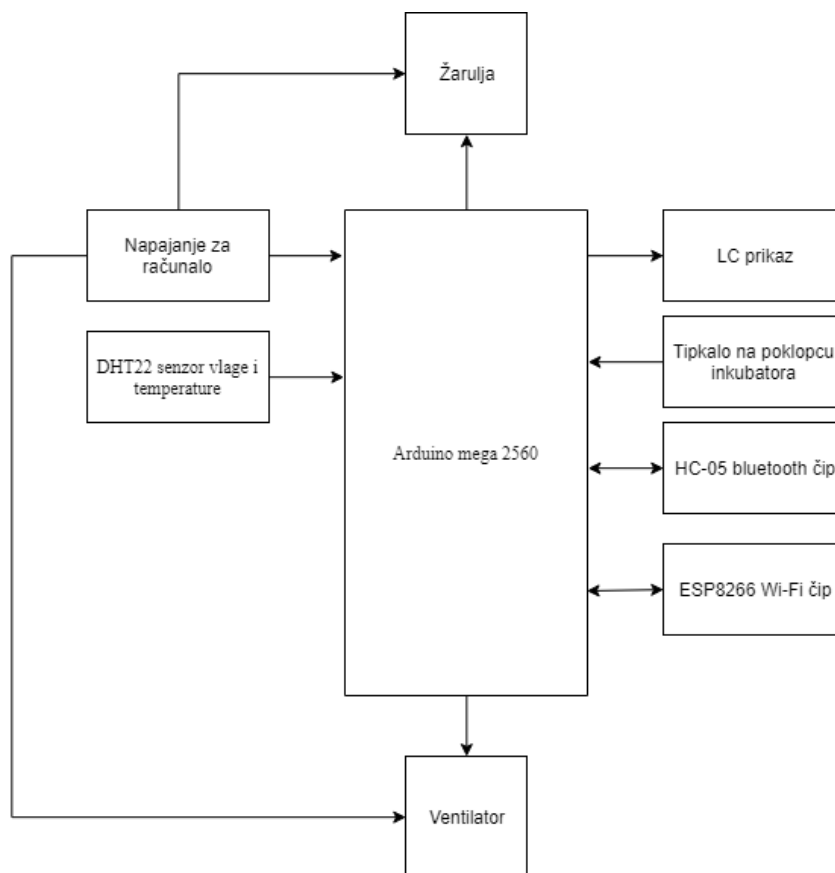
Slika 3.4. Strukturalni blok diagram sustava
