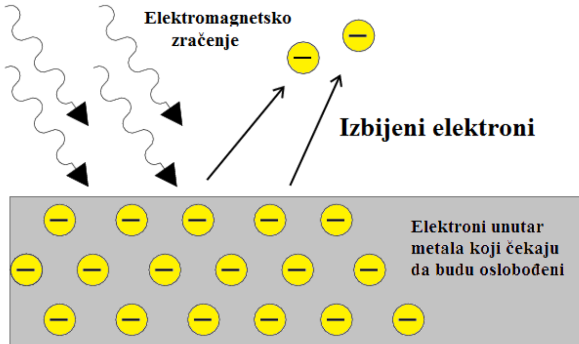
Slika 3.3.: Fotoelektrični efekt [22]
