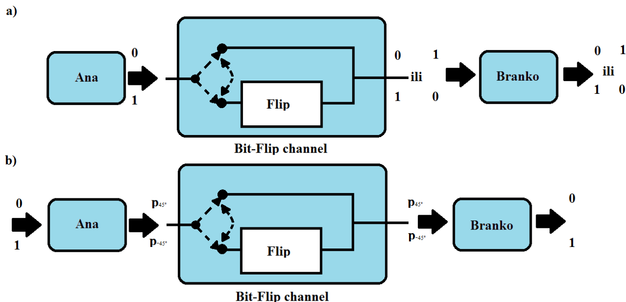
Slika 4.3.: Bit-Flip kanal [1]
