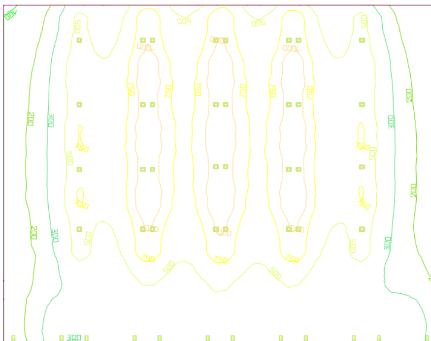
Slika 7.13. Prikaz rasvjetljenosti
