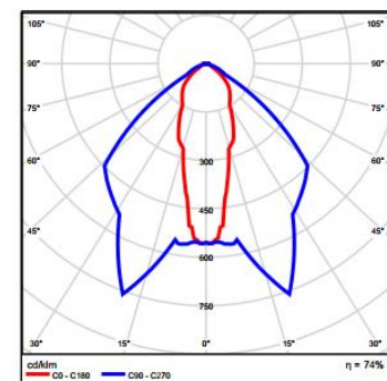
Slika 7.12. Disano 1158 JM-T
