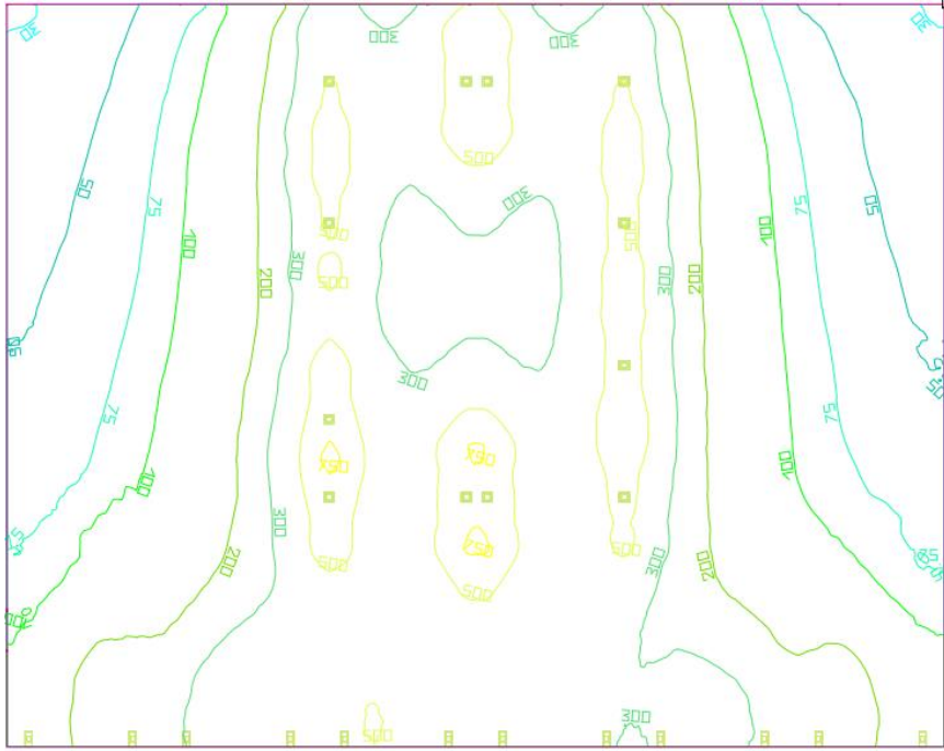
Slika7.15. Prikaz rasvijetljenosti
