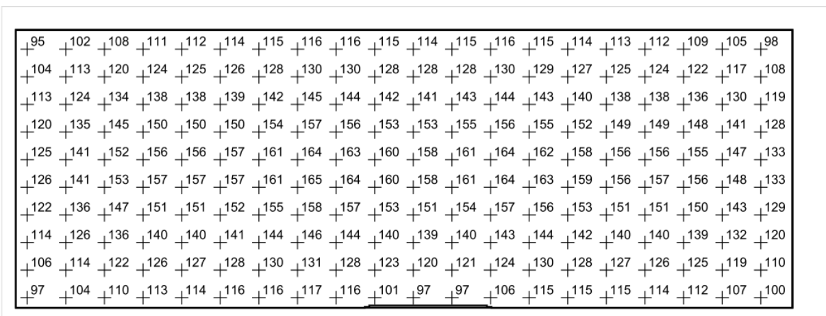
Slika 7.59. Brojčani prikaz rasvijetljenosti
