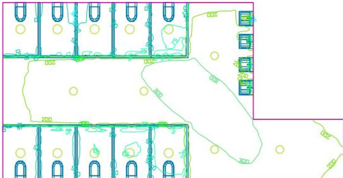
Slika 7.46. Prikaz rasvijetljenosti
