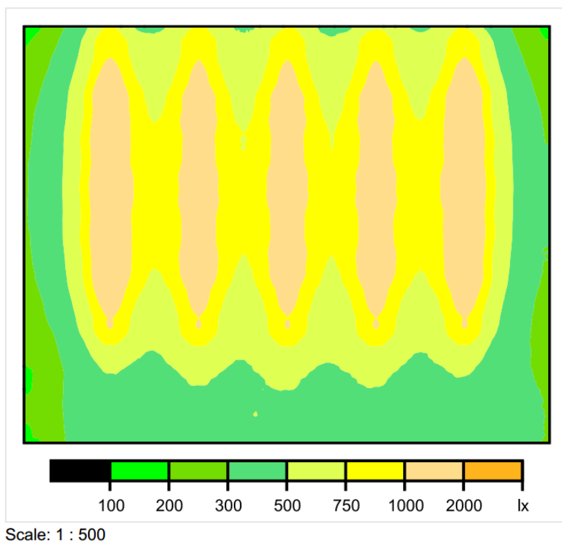
Slika 7.10. Grafički prikaz rasvijetljenosti
