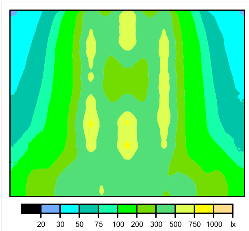
Slika 7.16. Grafički prikaz rasvijetljenosti
