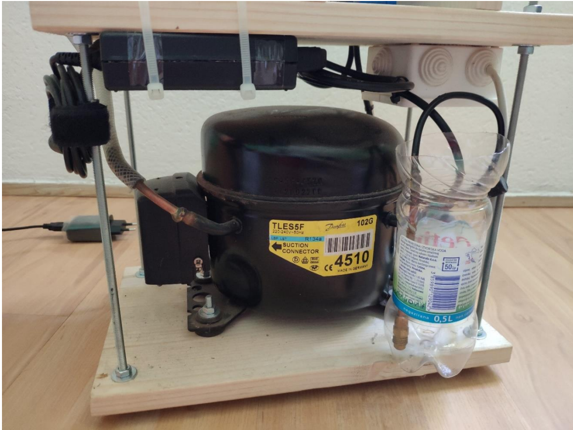
Slika 22. Ispuštanje kondenzata
