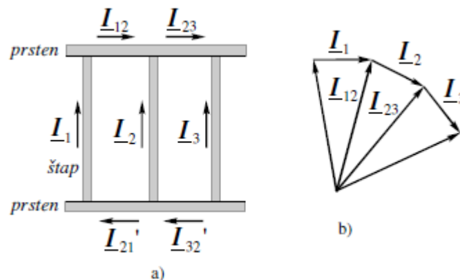
Slika 2.11. Struje u štapovima i prstenima kaveznog namota; a) struje u kavezu, b) fazorski prikaz
