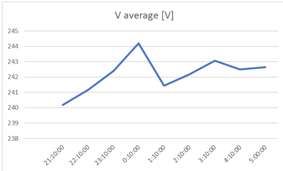
Slika 4.10. Grafikon mjerenja napona
