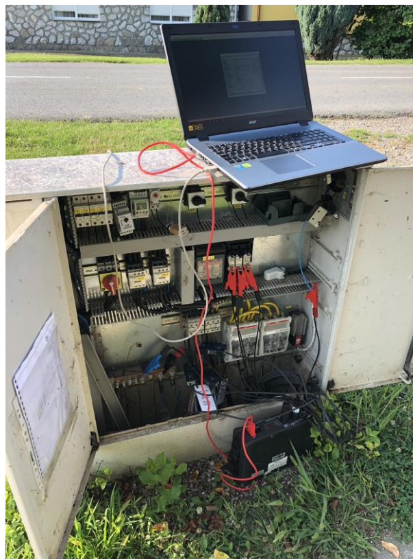
Slika 4.3. Upravljački ormar JR ispred ŽSTS 574
