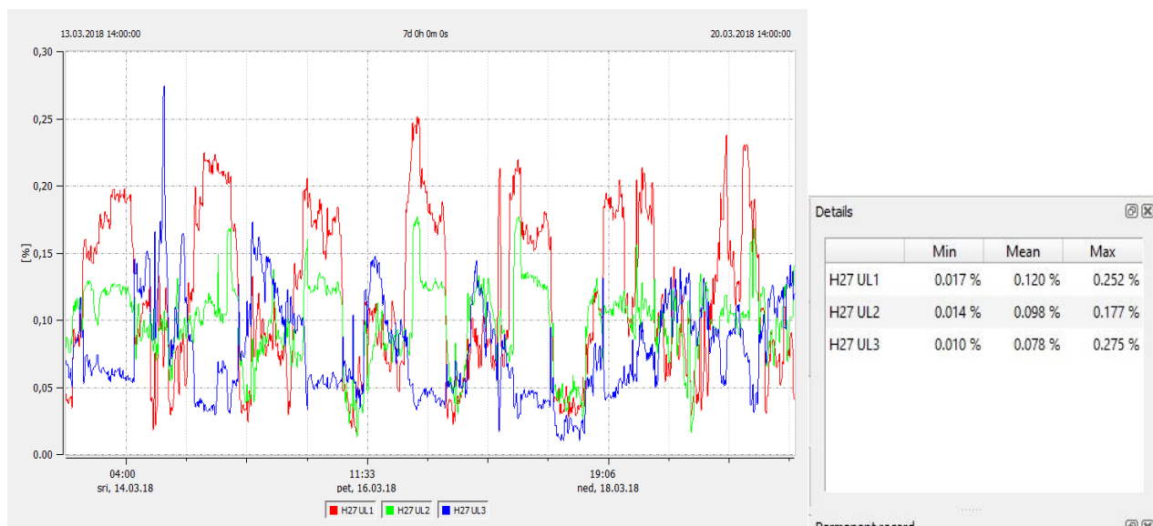
Slika 4.3. Analiza 27.harmonika
