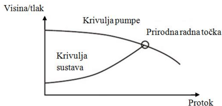
Slika 3.9. Kombinirane krivulje, [2]
