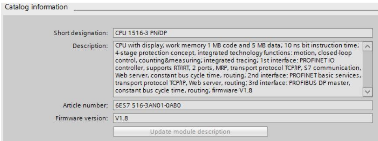
Slika 4.2. Karakteristike PLC_VT_S7-1516
