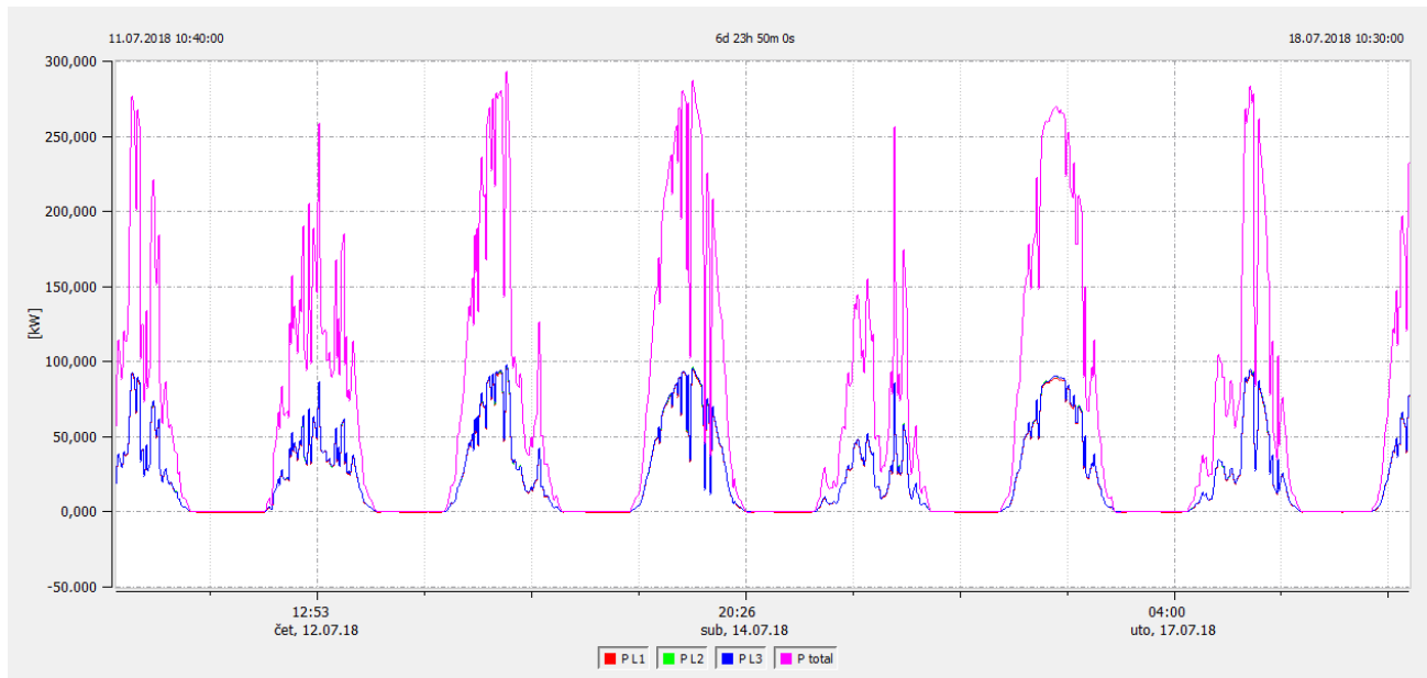
Slika 4.34. Predana trofazna radna snaga
