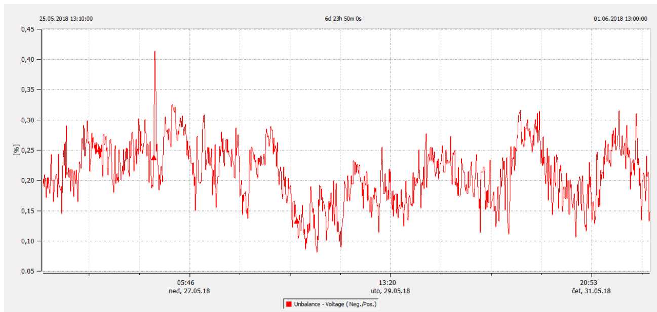
Slika 2.13. Nesimetrija napona
