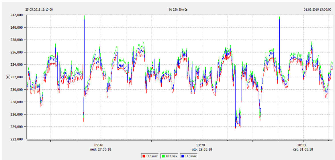
Slika 4.8. Maksimalne desetminutne efektivne vrijednosti napona
