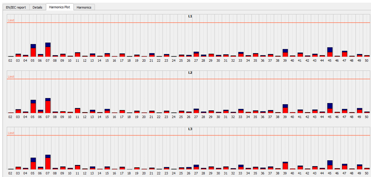
Slika 4.20. Detaljan prikaz vrijednosti viših harmonika
