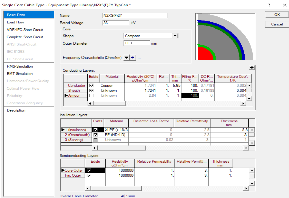
Slika 3.8 Uneseni svi parametri[6]
