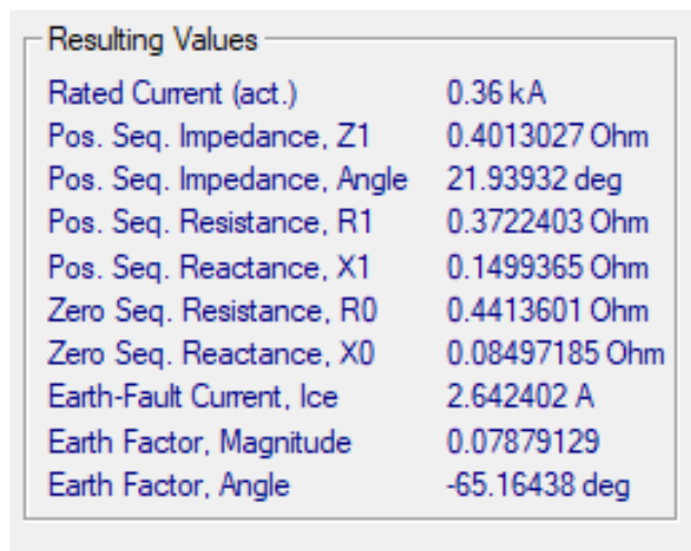
Slika 3.11. Rezultati proračuna za aluminij
