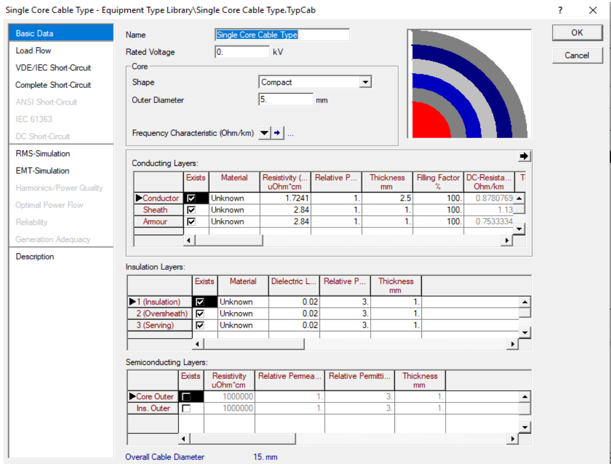
Slika 3.7. Početni prozor bez parametara[6]
