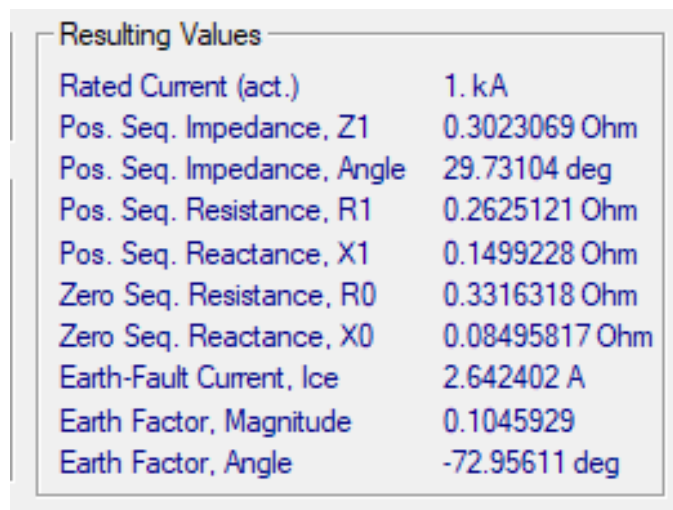
Slika 3.10 Rezultati proračuna za bakar
