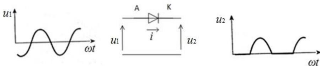
Slika 2.5. Dioda [2]
