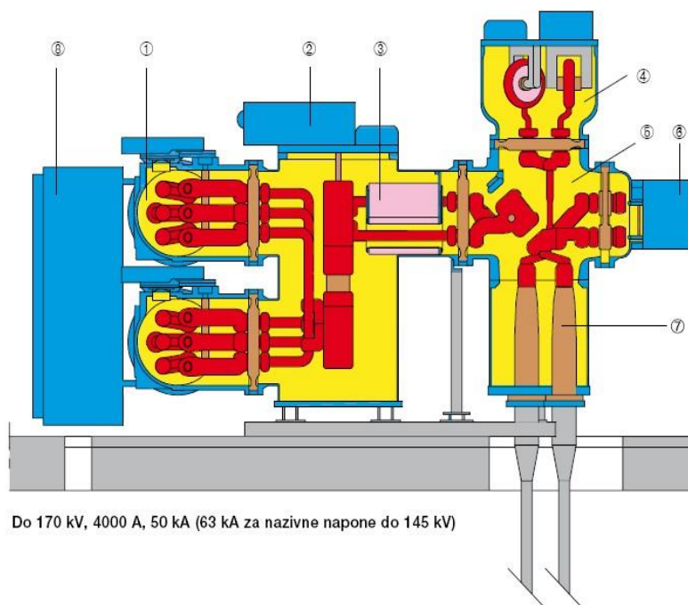
Slika 8.2 Primjer GIS postrojenja proizvodnje ABB[1]
