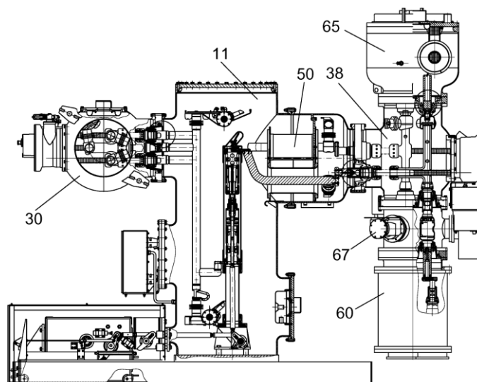
Slika 8.1 Primjer GIS postrojenja proizvodnje Končar[1]
