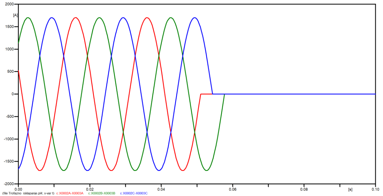
Sl. 4.5. Prikaz struja kroz prekidače.
