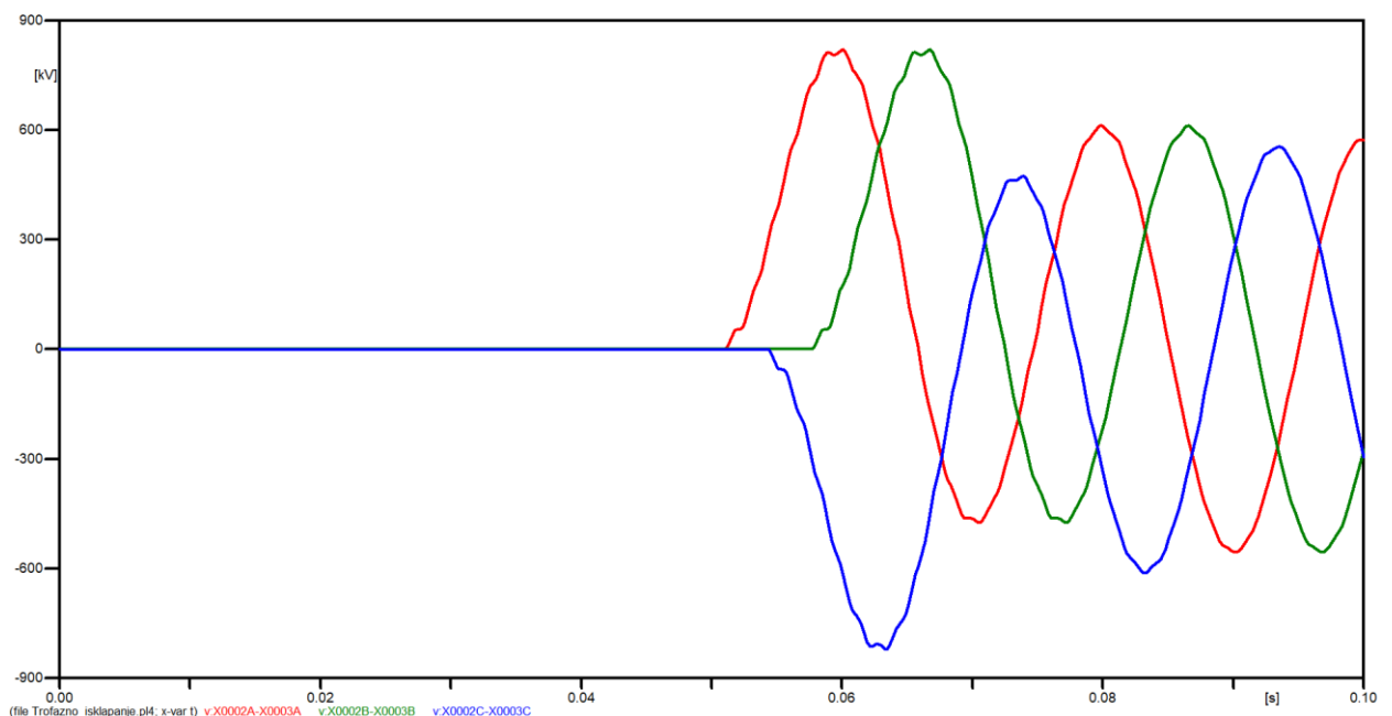
Sl. 4.6. Prenaponi na kontaktima prekidača.
