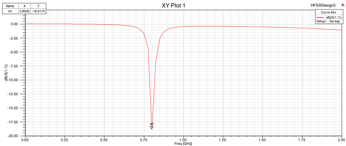
4.2.2.13. slika S_{11} parametra metamaterijalne antene
