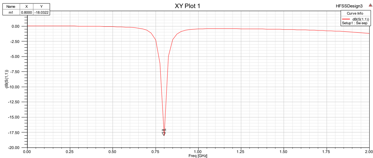
4.2.2.9. slika S_{11} parametra metamaterijalne antene
