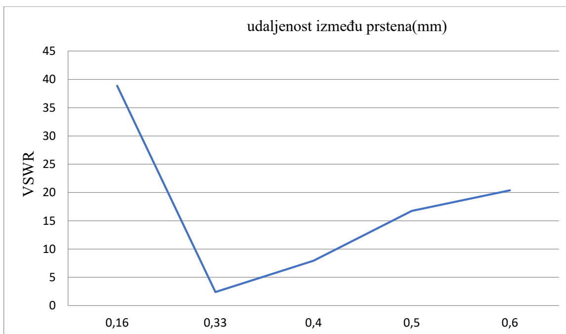
4.2.1.2. grafikon ovisnosti parametra VSWR o duljini razmaka između prstena
