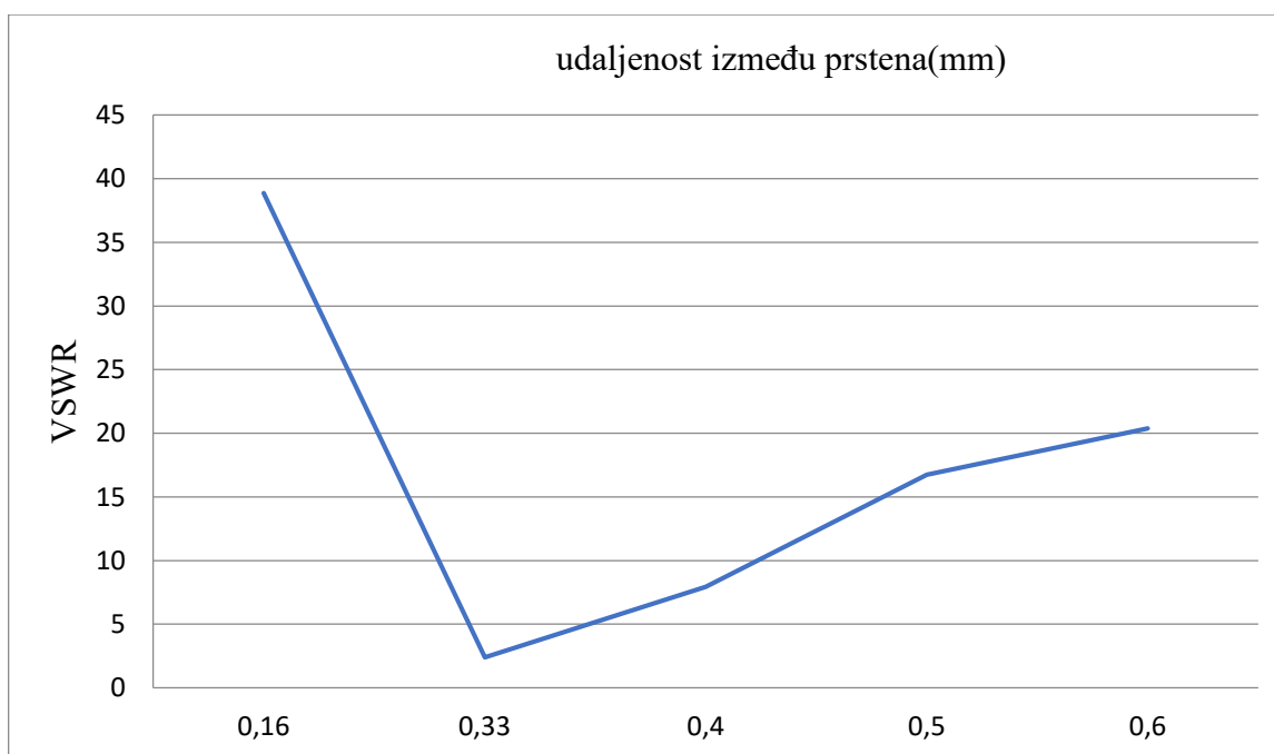
4.2.1.2. grafikon ovisnosti parametra VSWR o duljini razmaka između prstena
