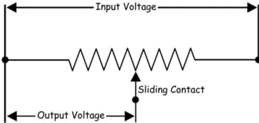
Slika 6.3. Prikaz potenciometra [10]
