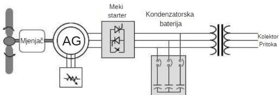
Slika 3.5. Tip 2 – Asinkroni generator s namotanim rotorom i kliznim prstenima [11]
