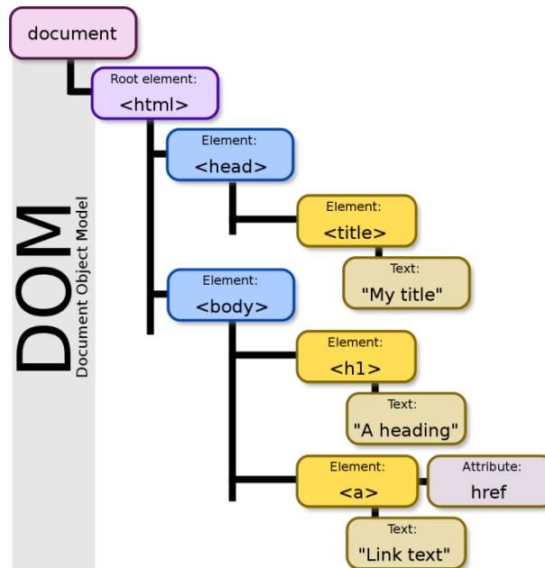
Sl. 2.2. Prikaz DOM strukture
