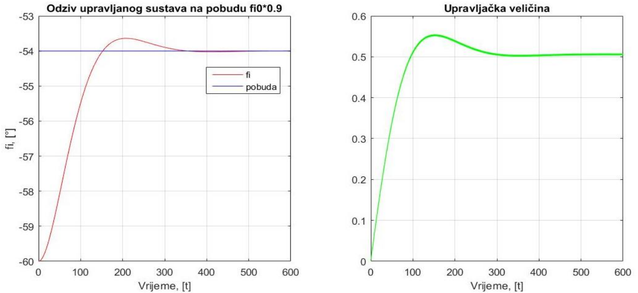
Slika 5.4. Odziv procesa upravljanog PID regulatorom na pobudu 0.9\varphi_0 .
