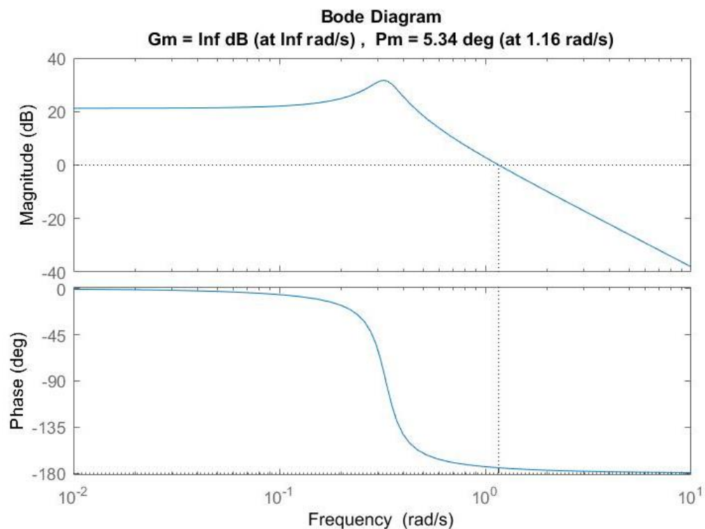
Slika 3.1. Bodeov dijagram za proces 2. reda
