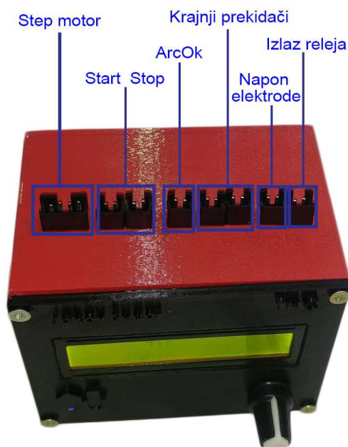
Slika 4.2. Povezivanje konektora
