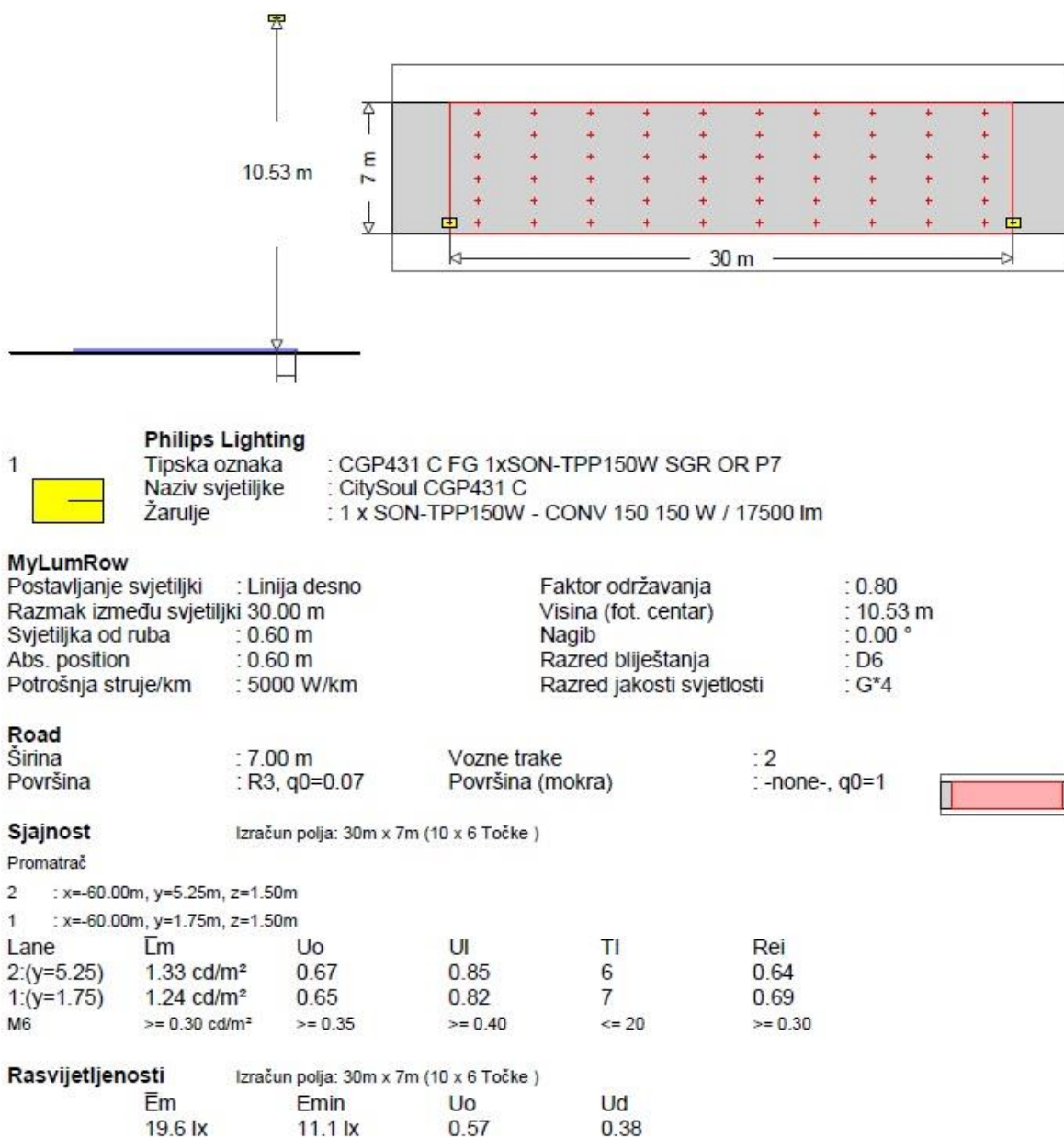
Slika 4.10. Rezultati simulacije.
