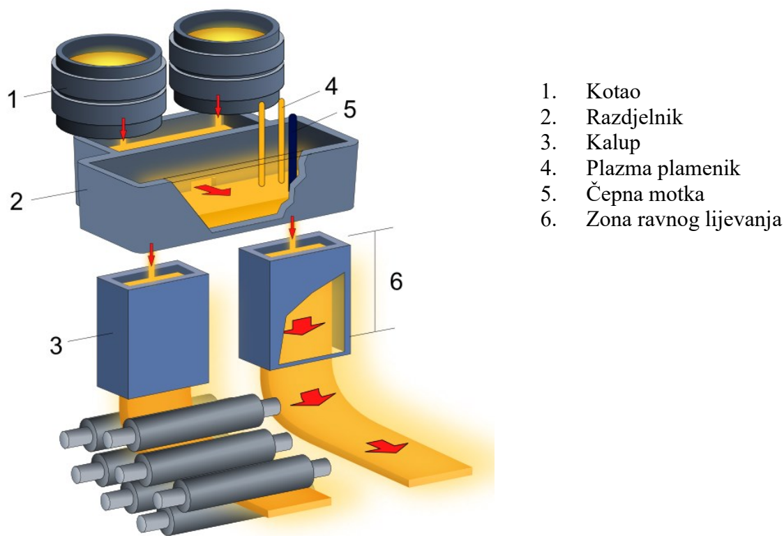
Sl. 2.6. Kontinuirano lijevanje (zакrivljeni, višekalupna izvedba).
