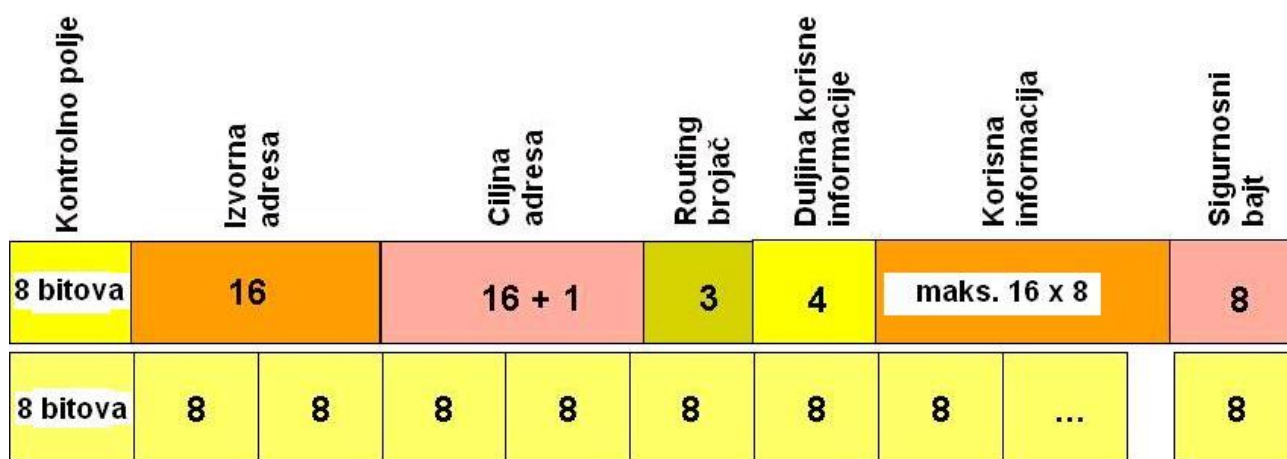
Slika 3.8. Struktura telegrama [5]
