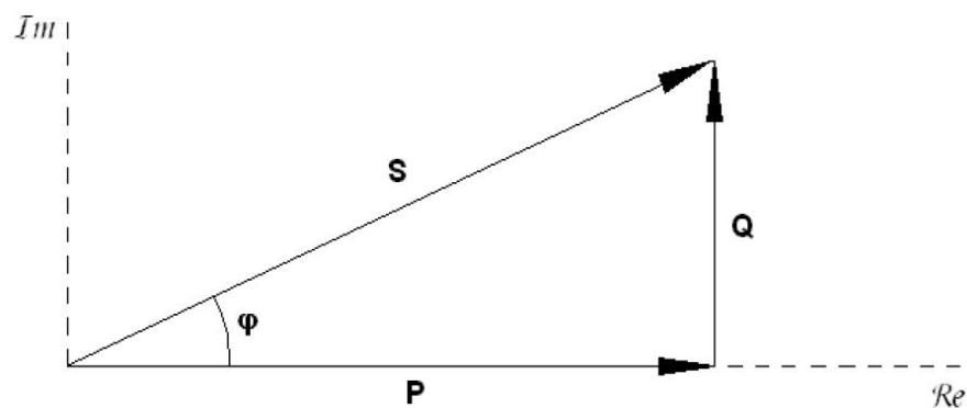
Sl. 2.1. Vektorski prikaz snaga.
