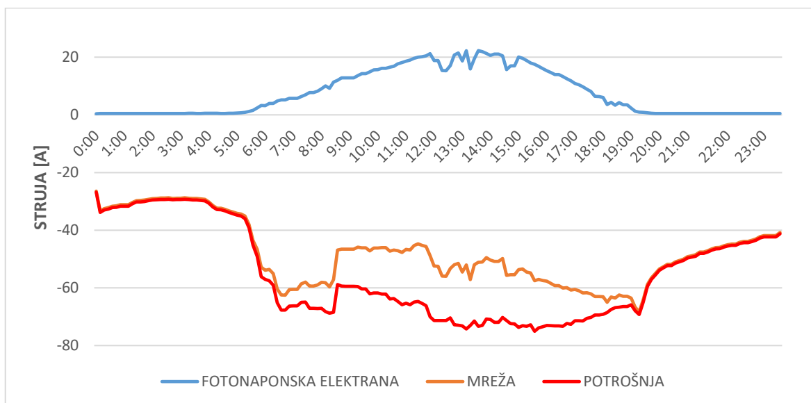
Slika 5.26. Promjena toka struje za sunčan dan
