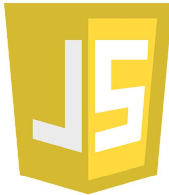
Slika 2.2. JavaScript logo
