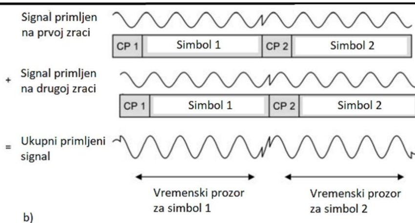
Sl.3.8. a) razlika između zaštitnog i cikličkog perioda b) princip rada cikličkog prefiksa na jednom podnositelju
