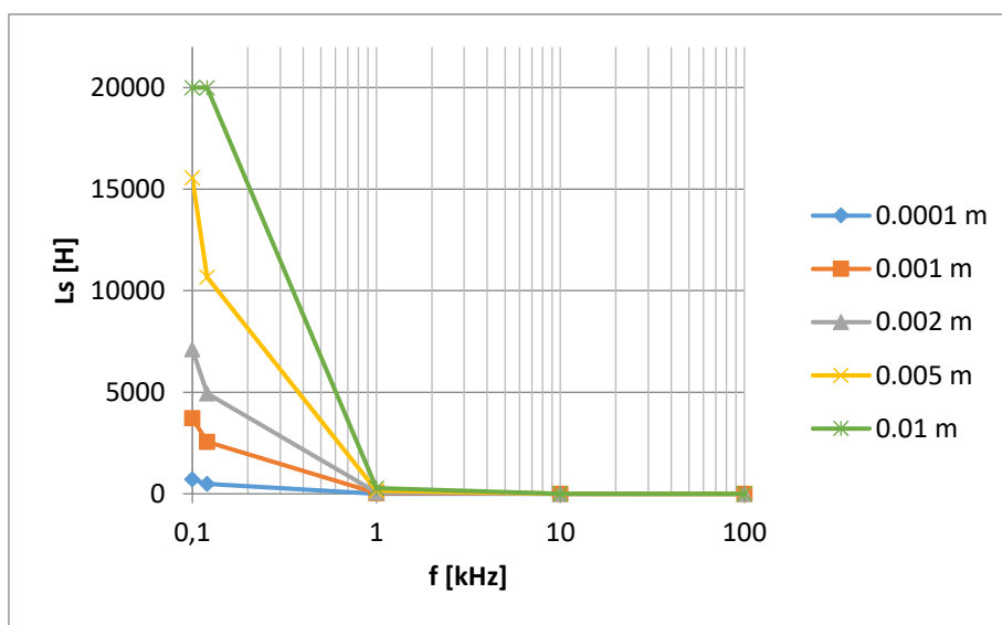
Slika 48. Serijski induktivitet L_s pločastog kondenzatora sa termoplastičnom folijom kao dielektrikom izmjeren UT612 uređajem
