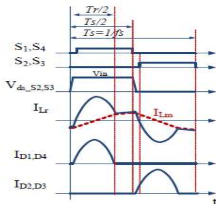
Slika 2.15. Valni oblici struja pri fs < fr .
