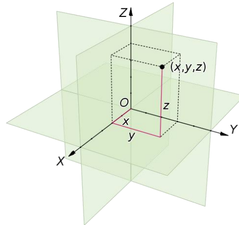
Skica 2.3.: Trodimenzionalni Kartezijev koordinatni sustav
