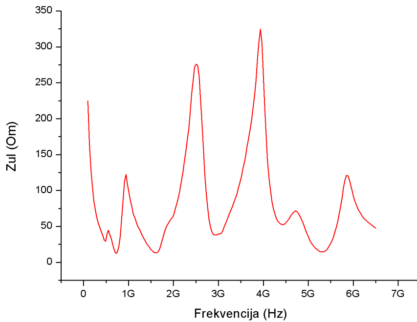
Slika 4.9. Ulazna impedancija
