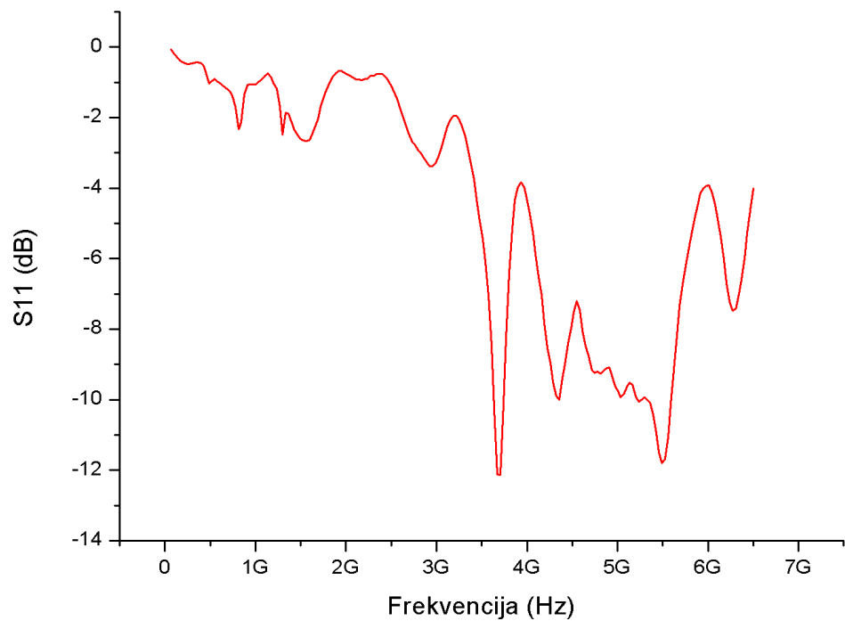
Slika 7.17. S11 Parametar
