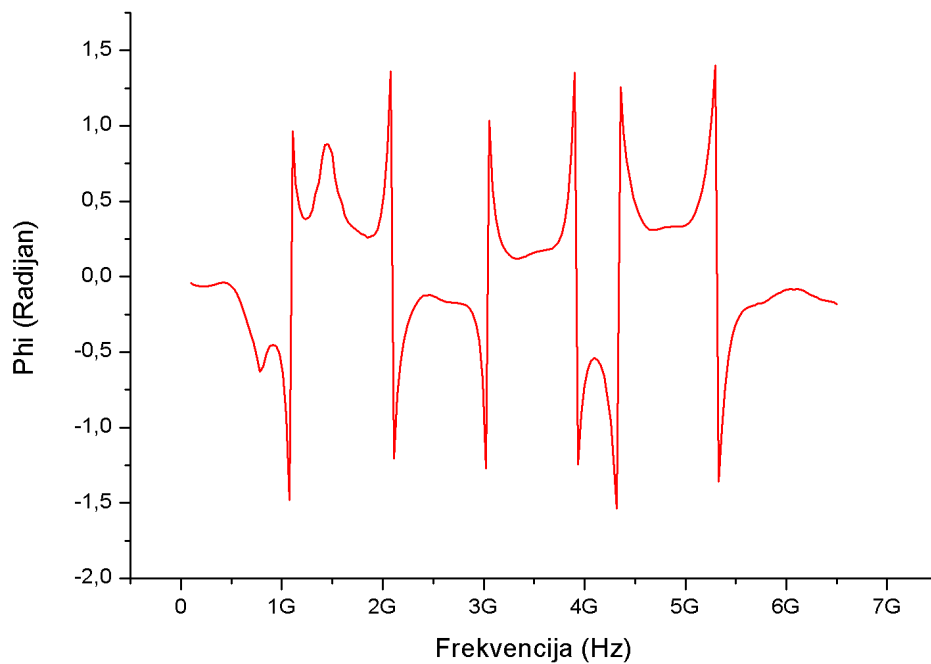
Slika 8.10. Fazni kut
