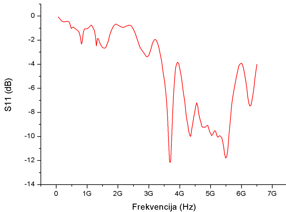
Slika 7.17. S11 Parametar
