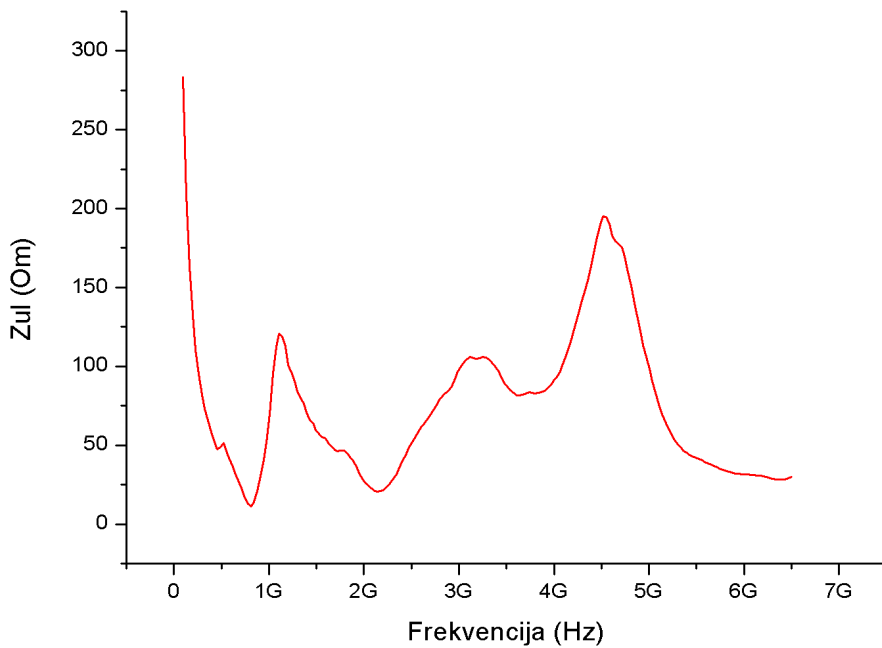
Slika 3.14. Ulazna impedancija
