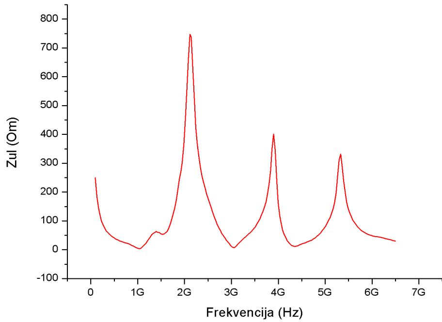
Slika 8.14. Ulazna impedancija
