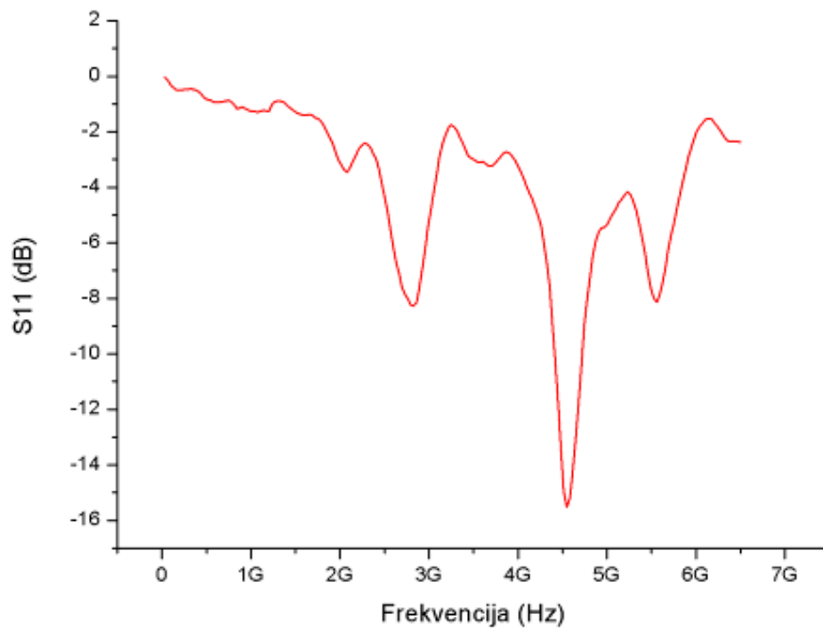
Slika 5.17. S11 Parametar
