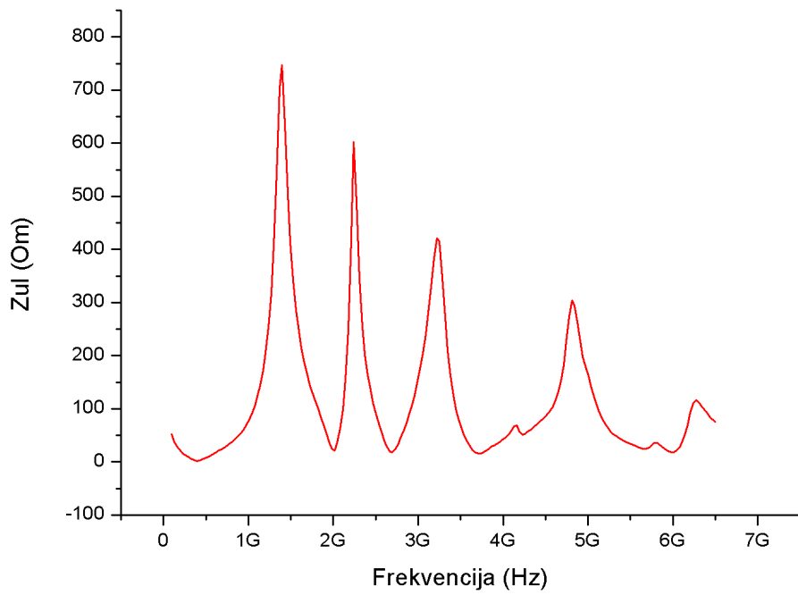
Slika 5.29. Ulazna impedancija
