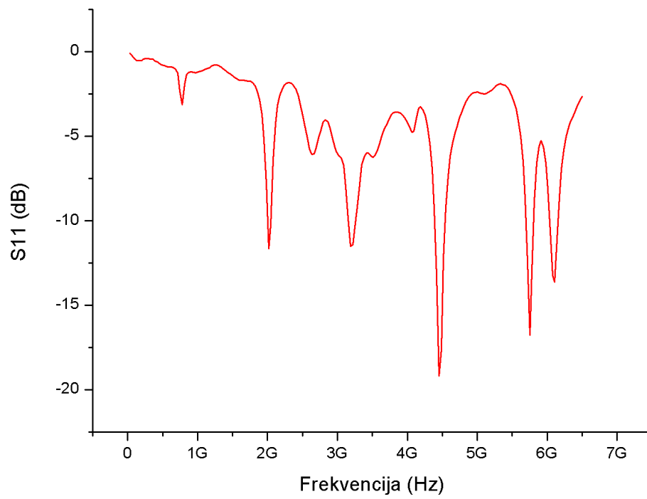
Slika 5.22. S11 Parametar
