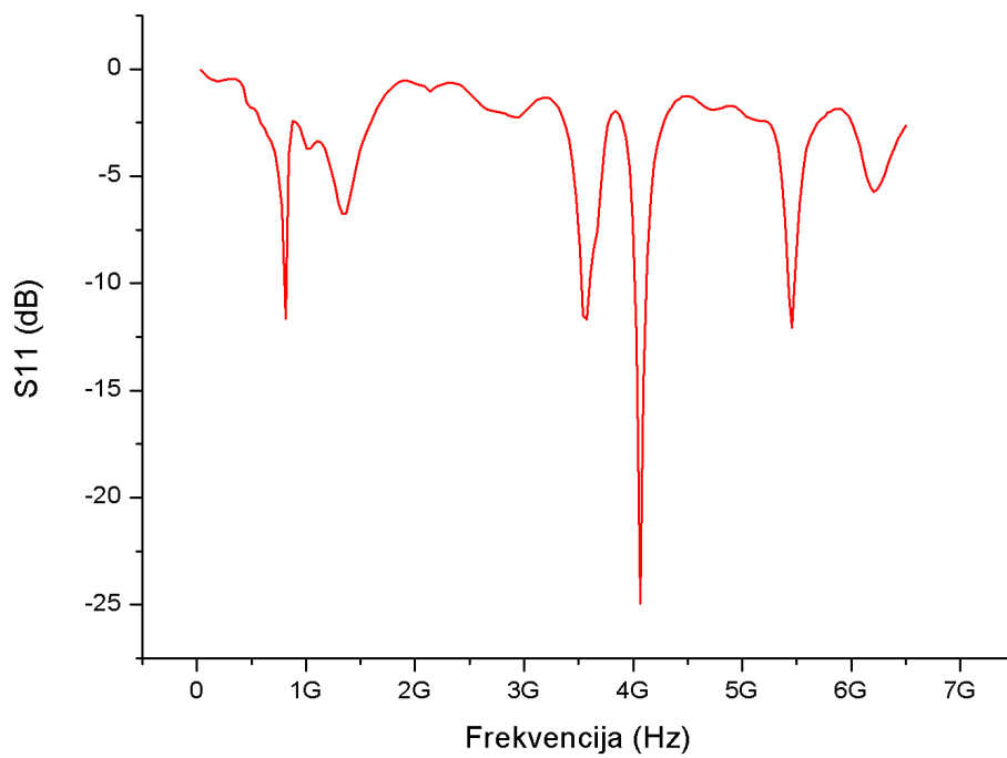
Slika 6.27. S11 Parametar
