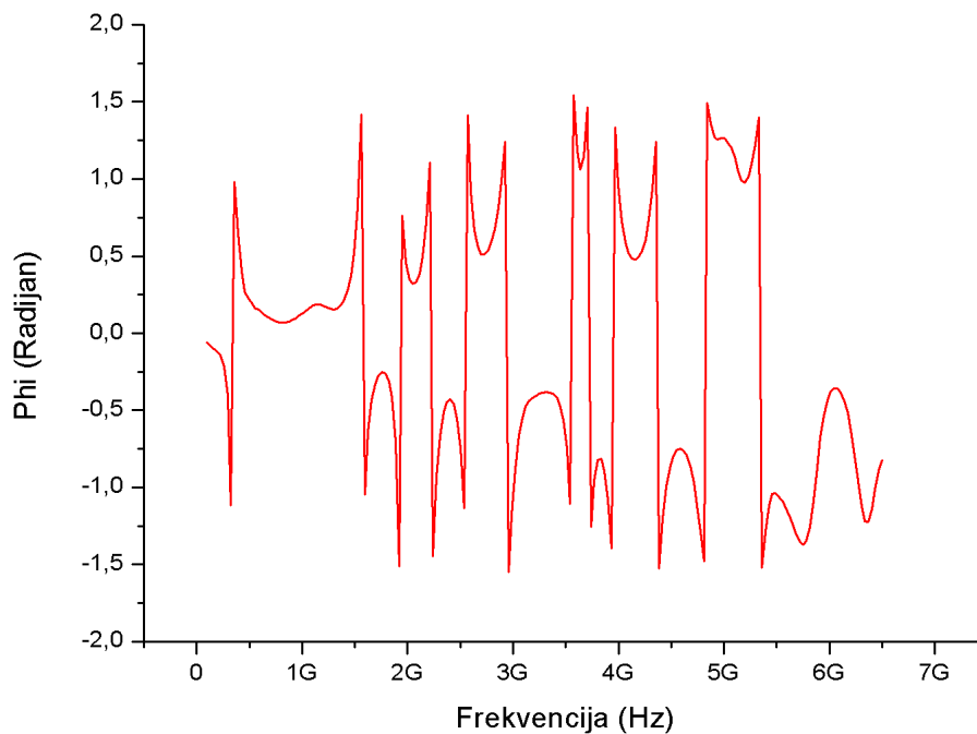
Slika 3.30. Fazni kut
