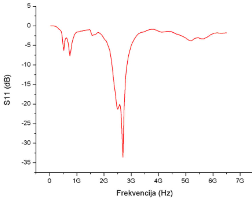
Slika 6.2. S11 Parametar
