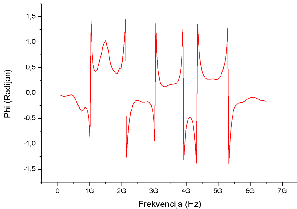
Slika 8.15. Fazni kut
