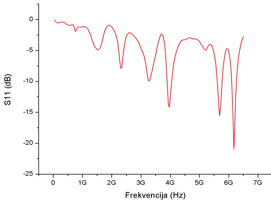
Slika 7.22. S11 Parametar
