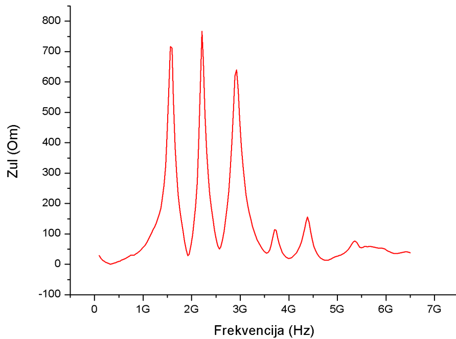
Slika 3.24. Ulazna impedancija
