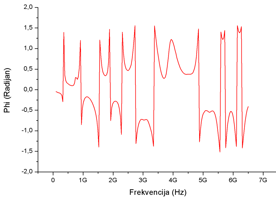
Slika 7.25. Fazni kut
