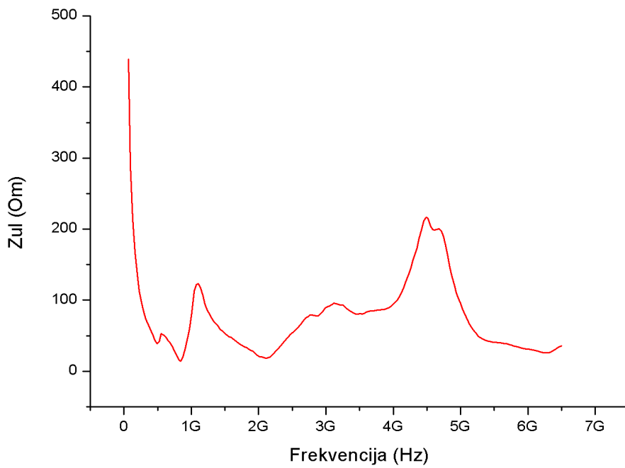
Slika 3.4 Ulazna impedancija
