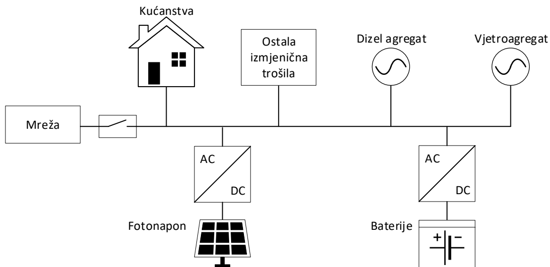
Slika 2.9. Izmjenična mikromreža [13]
