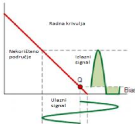
Slika 3.9. Radna krivulja klase AB pojačala
