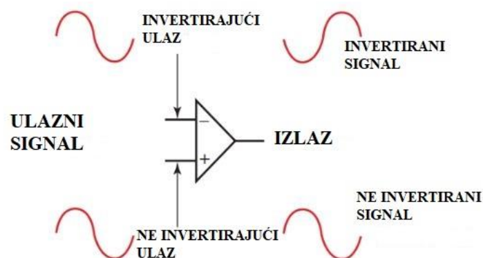
Slika 2.5. Operacijsko pojačalo
