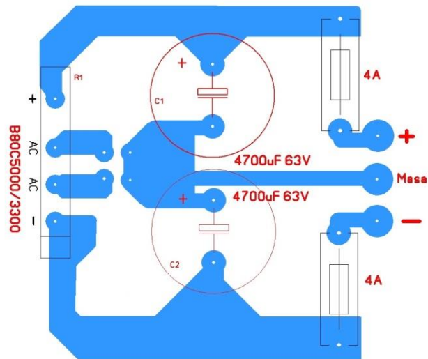
Slika 4.1. Montažna shema ispravljaja
