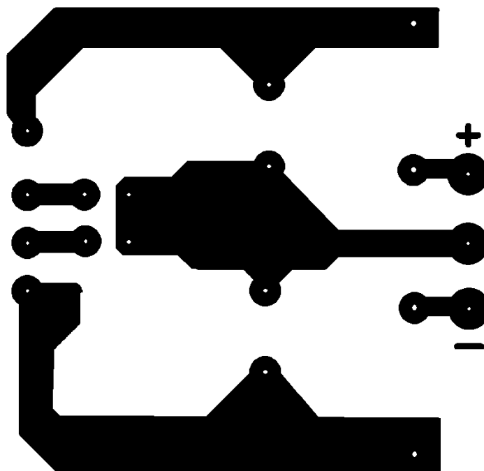
Slika 4.4. Shema tiskanih vodova ispravljачa
