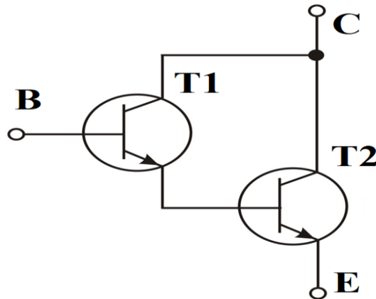
Slika 2.4. Darlingtonov spoj
