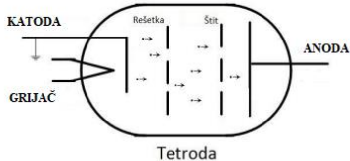
Slika 3.2. Tetroda
