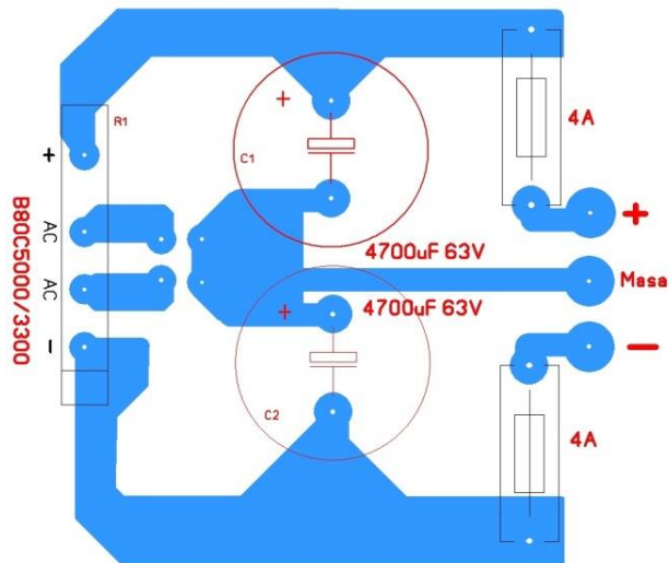
Slika 4.1. Montažna shema ispravljča
