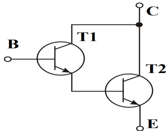
Slika 2.4. Darlingtonov spoj
