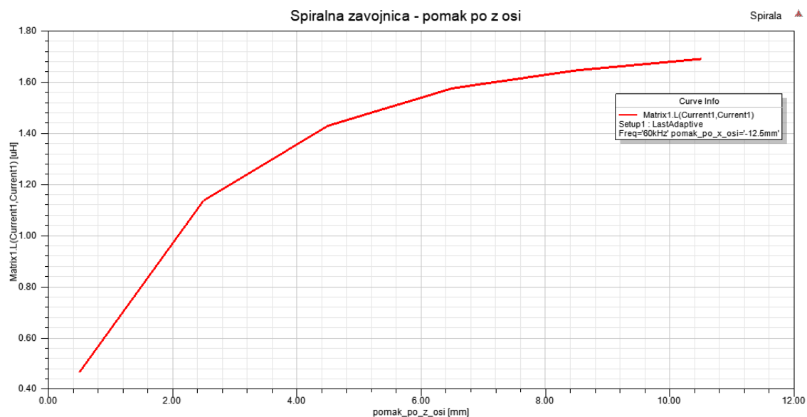
Slika 5.12. Promjena induktiviteta pomakom po z osi
