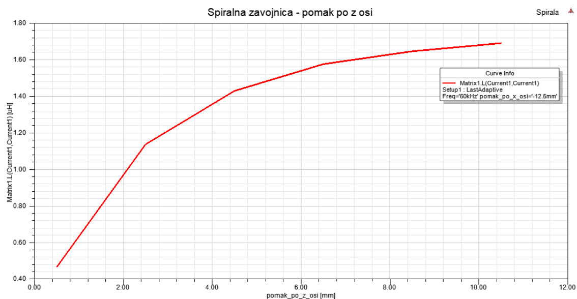
Slika 5.12. Promjena induktiviteta pomakom po z osi
