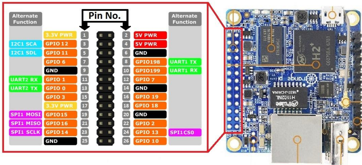
Slika 2.2. Orange Pi Zero GPIO
