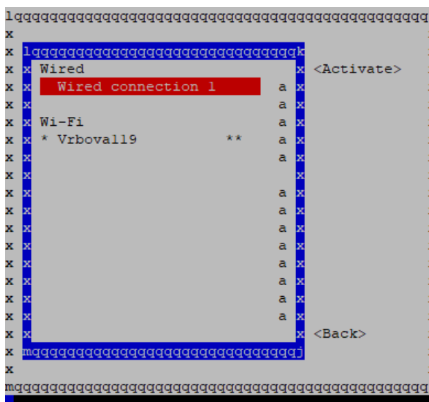
Slika 3.10.Odabir načina povezivanja
