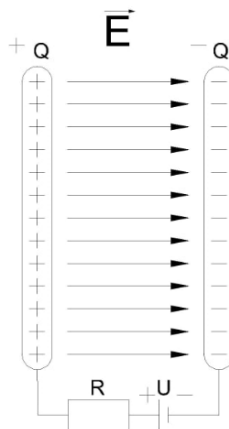
Slika 3. 3. Shema pločastog kondenzatora. [17]
