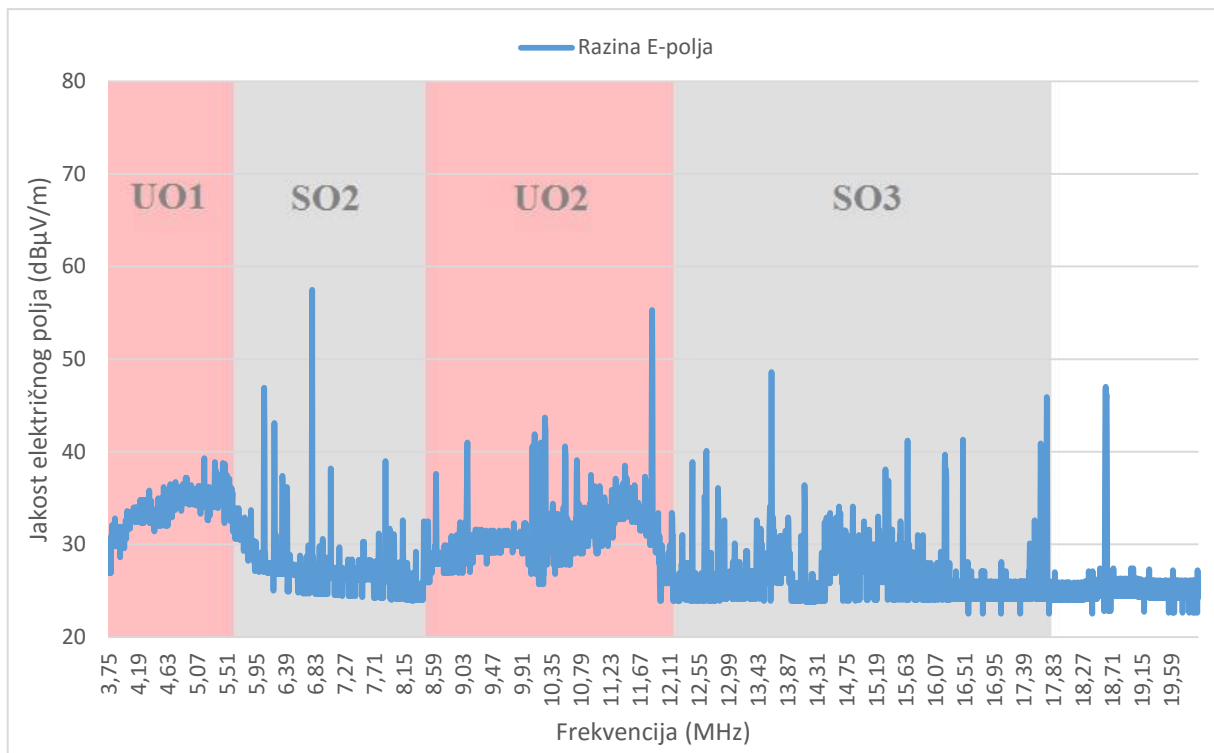
Slika 7.7. Vrijednosti izračenog električnog polja u frekvencijskom opsegu od 3,75 MHz do 20 MHz za jednog korisnika, balansirana parica, na udaljenosti 3 m od kabela
