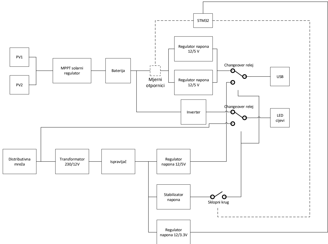
Slika 4. 1Blok dijagram
