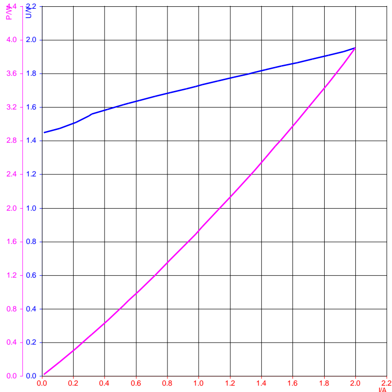
Slika 3.10. Karakteristika elektrolizatora
