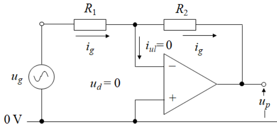
Slika 3.4. Invertirajuće pojačalo [9]
