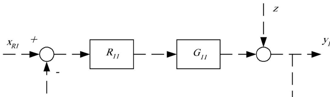
Slika 2.2. Utjecaj sprege na prvu regulacijsku stazu.
