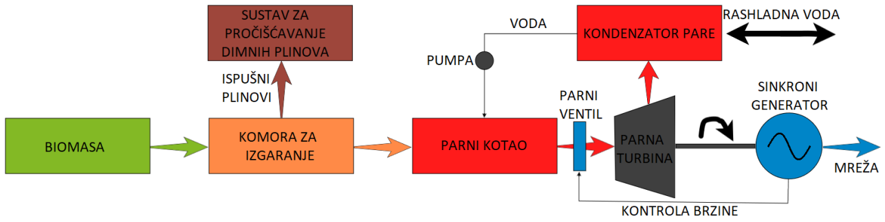
Slika 3.3. Pojednostavljena shema elektrane na biomasi [16]
