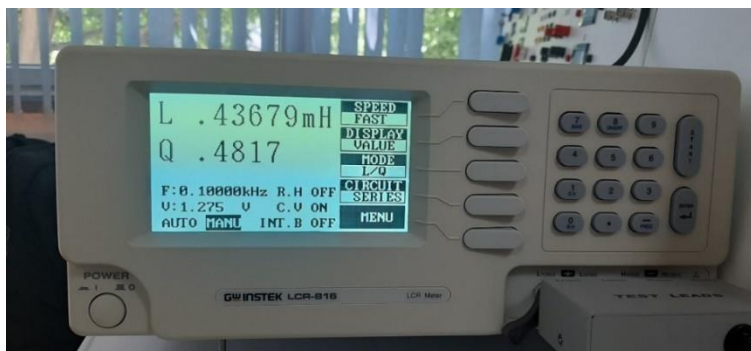
Slika 4. 14. Postavke instrumenta pri mjerenju zavojnice nazivnog induktiviteta 0,45[mH].
