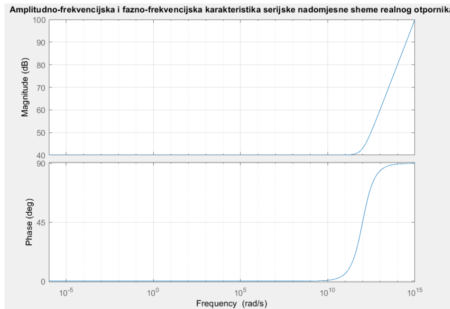
Slika 3. 14. Amplitudno-frekvencijska i fazno-frekvencijska karakteristika serijske nadomjesne sheme realnog kondenzatora.
